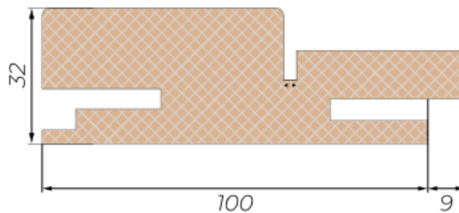
DETALIU TOC REGLABIL MDF 10X32X2050
